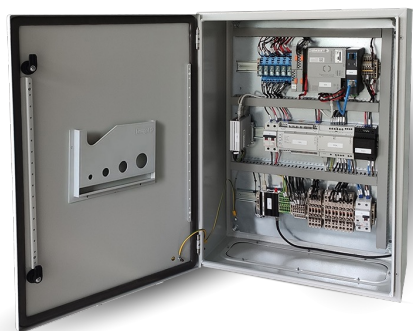
CONTROLLORE CENTRALE D'IMPIANTO
